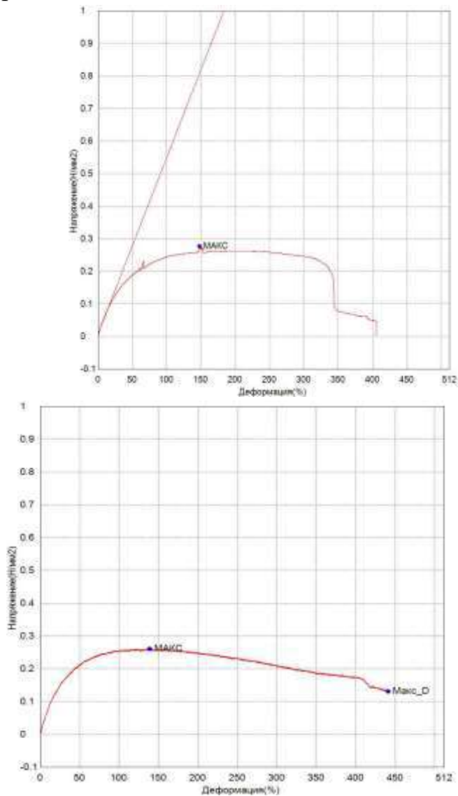
Рисунок 2а. Кривые напряжения-деформации БСК и олеогеля.
