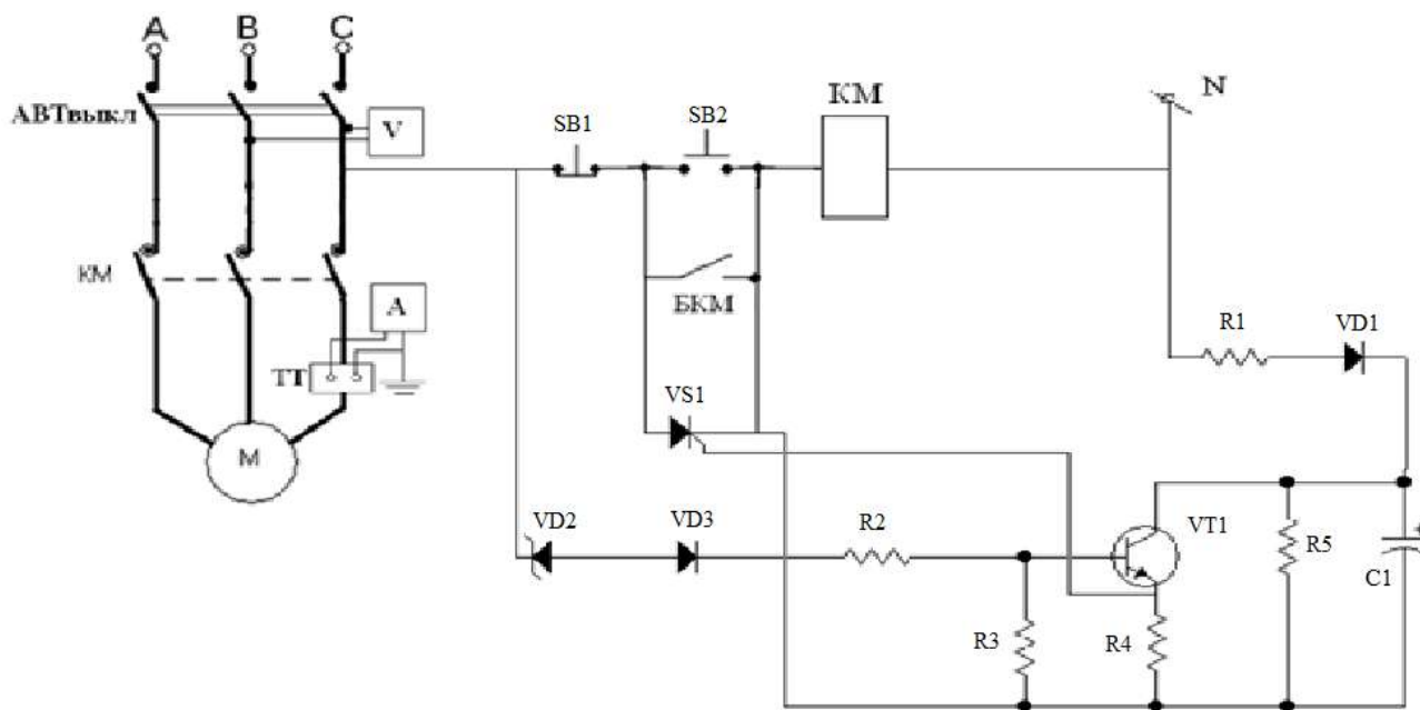
4-rasm. Nasos agregatini avtomatik qayta ulash prinsial blok sxemasi (AQU).
