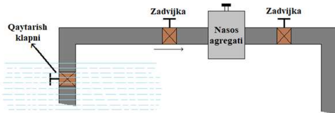
3-rasm. Qaytarish klapani orqali sug'orish tizimi.
