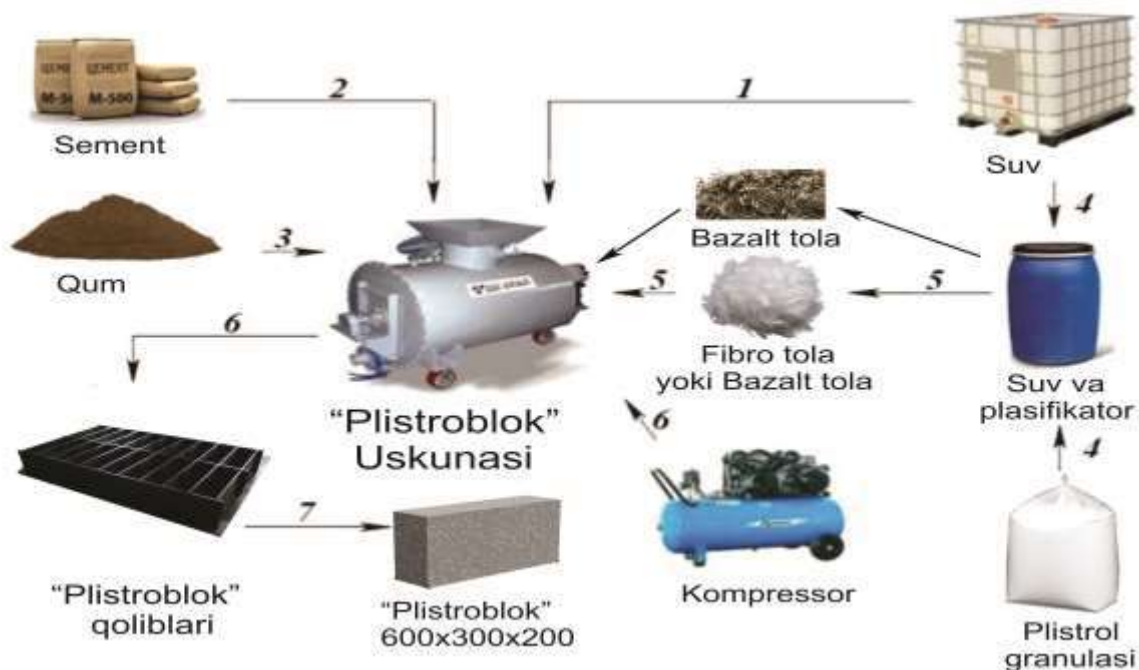
"Politsroblok"ni ishlab chiqarish jarayoni va asosiy vositalari.
