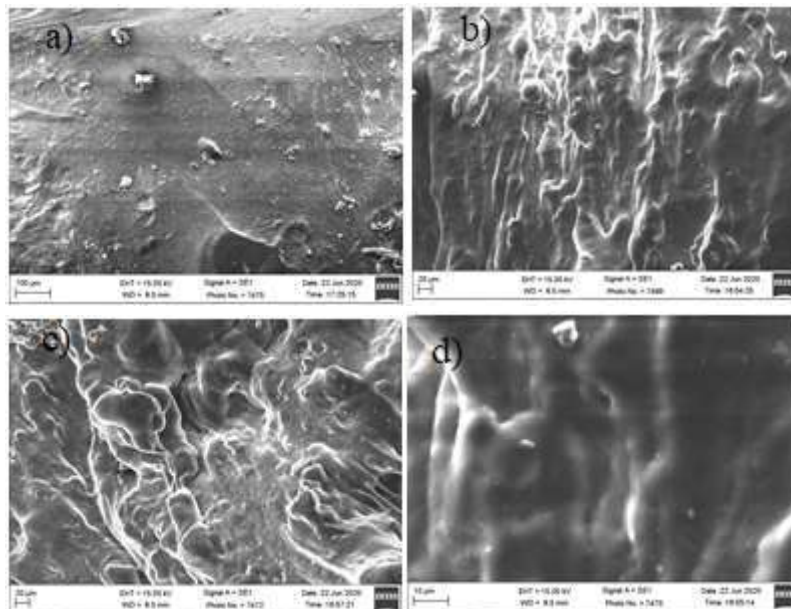
Рисунок 3. СЭМ-изображения СКИ (а), БСК (б), СКН (в), ТК (г).
