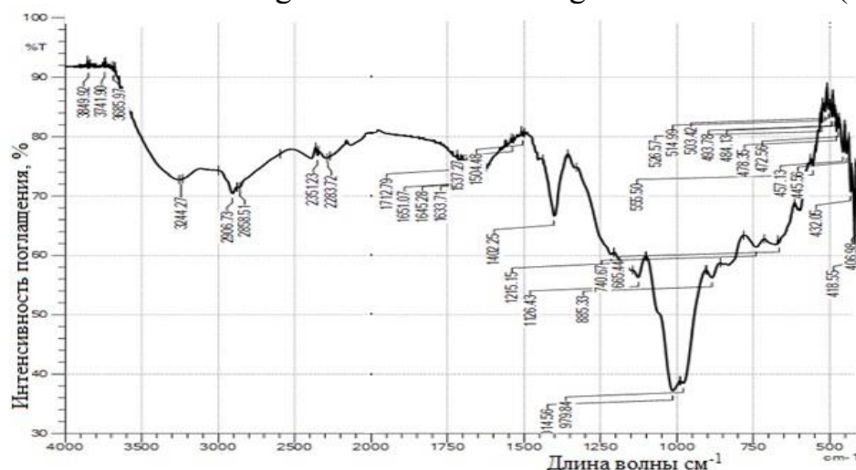
2-rasm. Oltiugurt, azot va fosfor saqlagan oligomerining IQ-spektri.
